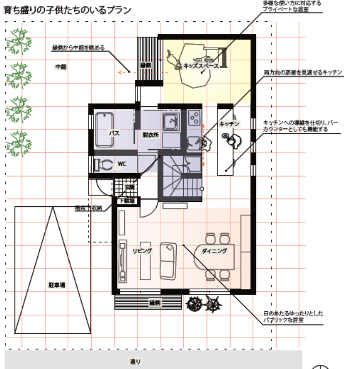
配置図兼1階平面図 S=1:100
